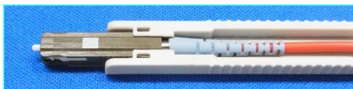
MUコネクタの装着
