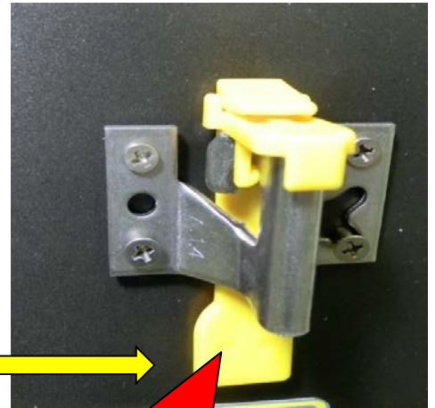
キャップ部
